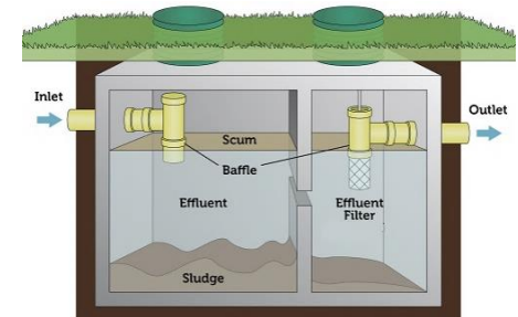
Tanque de aguas negras que funciona apropiadamente. La capa de suciedad y aguas residuales se guardan en el tanque.
